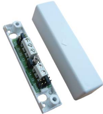
MST
