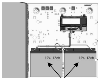
Umístění 2 x 12 V 17 nebo 18 Ah
