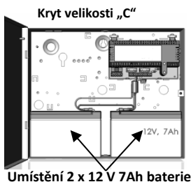
Umístění 2 x 12 V 7Ah baterie
