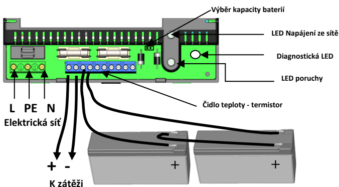
Obrázek 3 – zapojení
