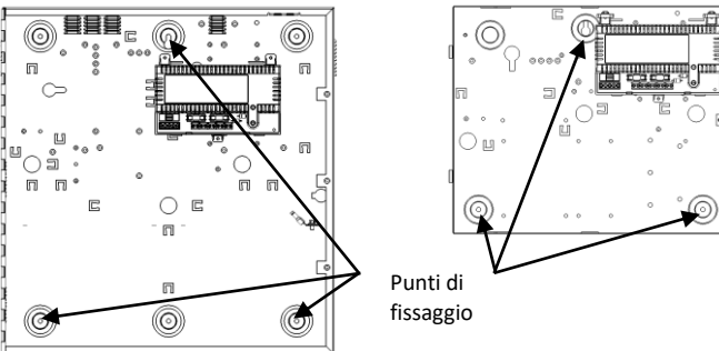
Figure 2 Posizionamento batterie
