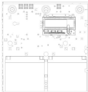
2402ST se skříní H a bateriemi 38Ah
