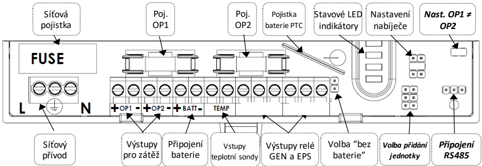
Obr. 4 – Rozložení svorek a volba režimů
