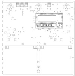
2402ST in contenitore H con batterie da 38Ah
