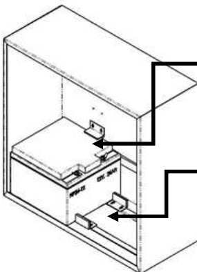
2402ST in contenitore H con batterie da 24Ah (batteria omessa per chiarezza)
