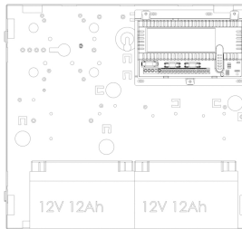
2402ST in contenitore K con batterie da 12Ah
