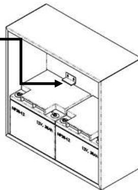
2402ST in contenitore H con batterie da 38Ah
