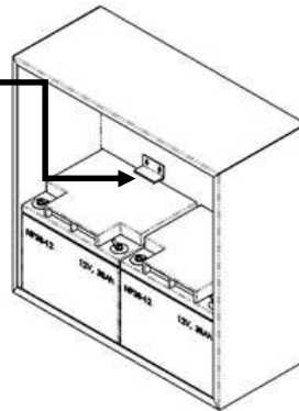
2402ST in H-Box mit 38-Ah-Batterien
