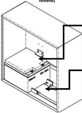
2402ST in H-Box mit 24-Ah-Batterien (Batterie zugunsten der Übersichtlichkeit fehlend)
