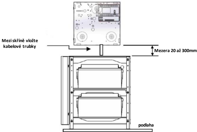
Obr. 3 – Skříně baterií (BATT-BOX-65)
