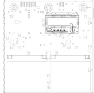
2405ST se skříní H a bateriemi 38Ah
