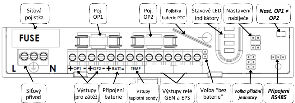
Obr. 4 – Rozložení svorek a volba režimu
