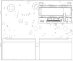
2405ST se skříní C a bateriemi 7Ah
