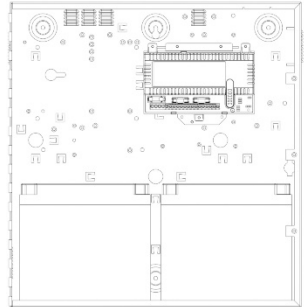
2405ST in E-Box mit 17-Ah-Batterien
